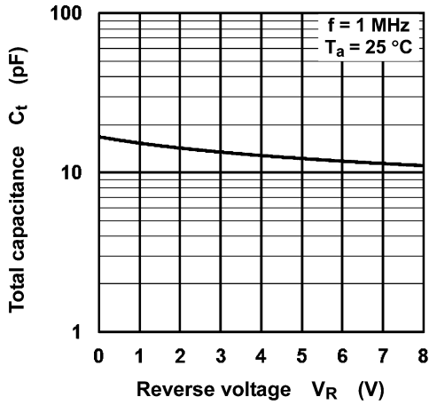
Fig. 8.3 C_t - V_R
