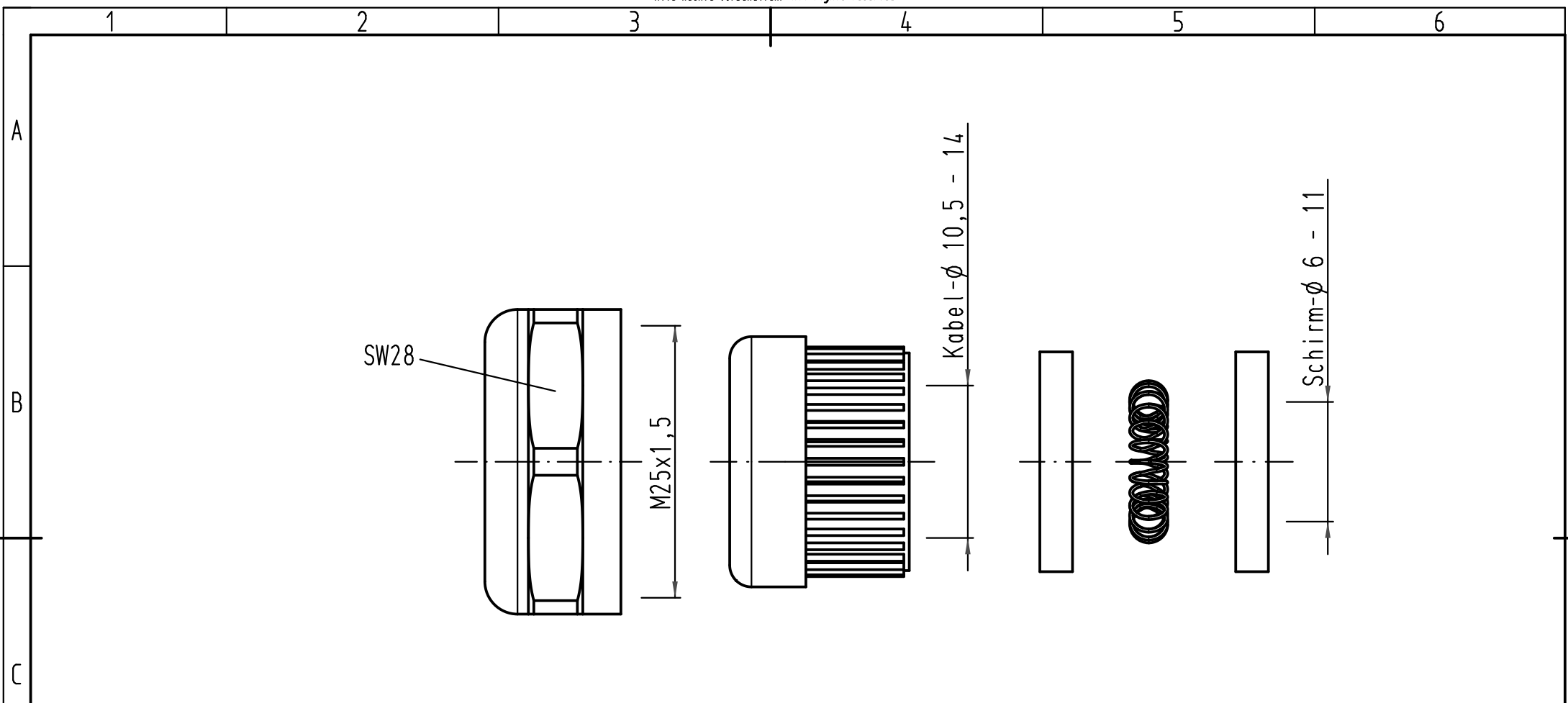
Für EMV Tüllengehäuse - Metall for EMC hoods - metal
