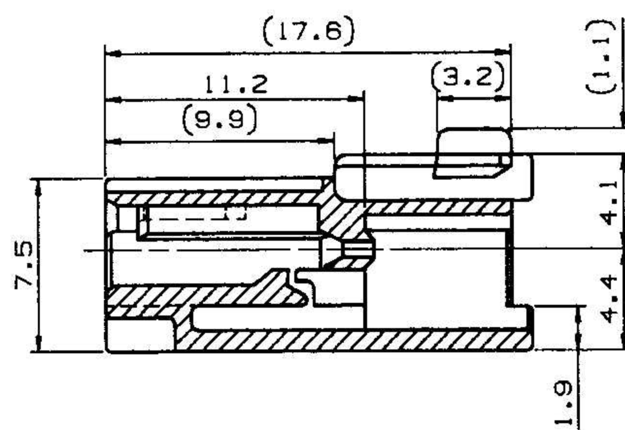
断面 A-A (SECT. A-A)
