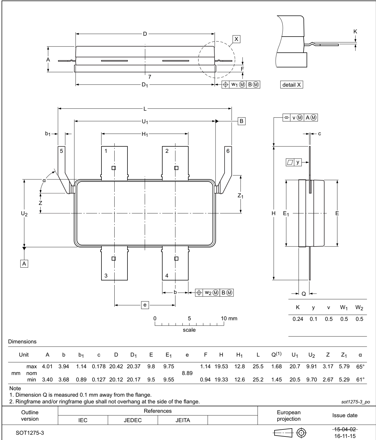
Fig 21. Package outline SOT1275-3
