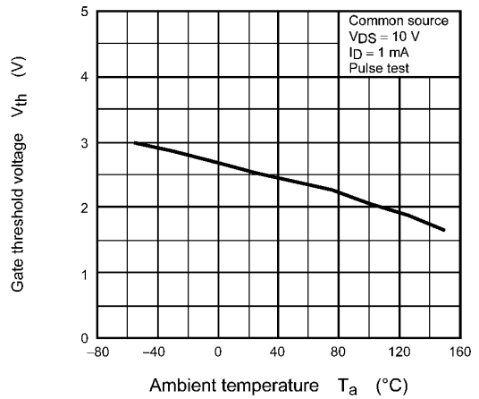
Fig. 8.10 V_{th} - T_a
